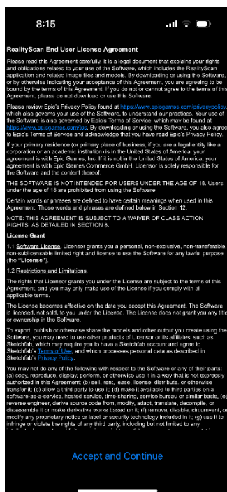
Obr. 8 Licenčné podmienky
