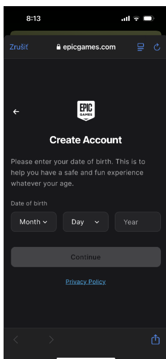
Obr. 4 Dátum narodenia
