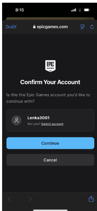
Obr. 7 Potvrdenie účtu
