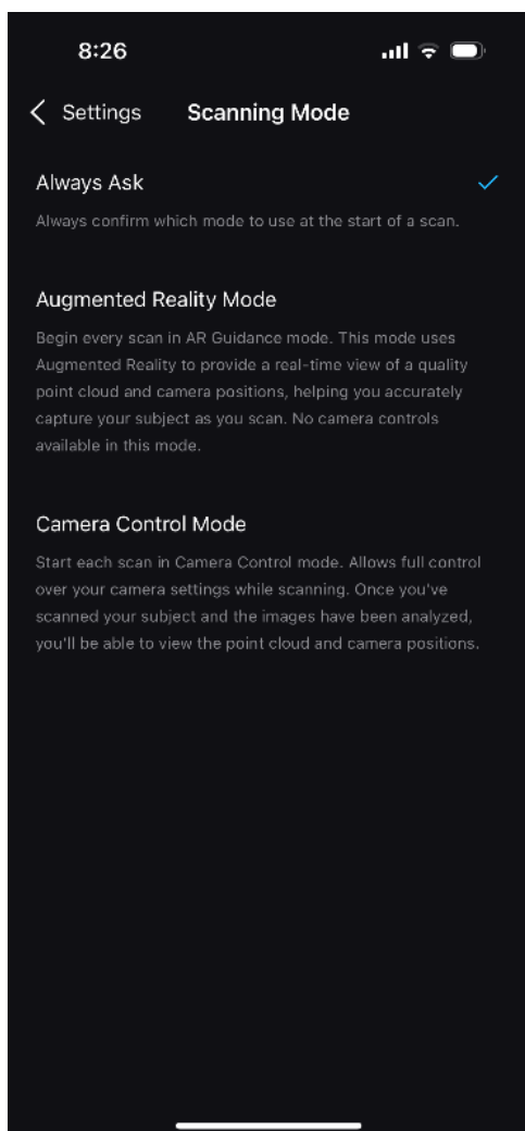
Obr. 12 Módy skenovania
