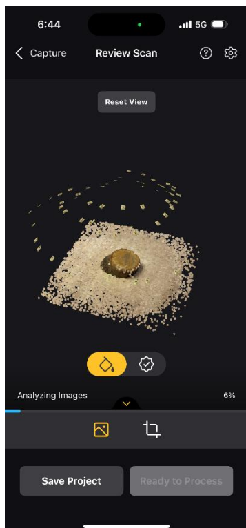
Obr. 19 Analyzovanie fotografií
