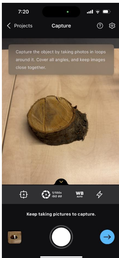
Obr. 16 Zachytenie objektu
