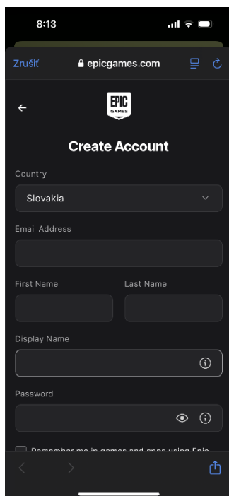
Obr. 5 Formulár
