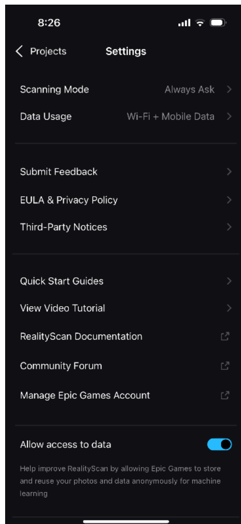
Obr. 11 Nastavenia
