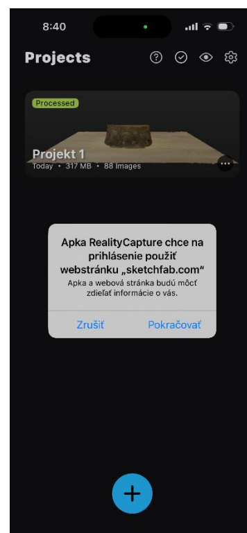
Obr. 30 Prihlásenie
