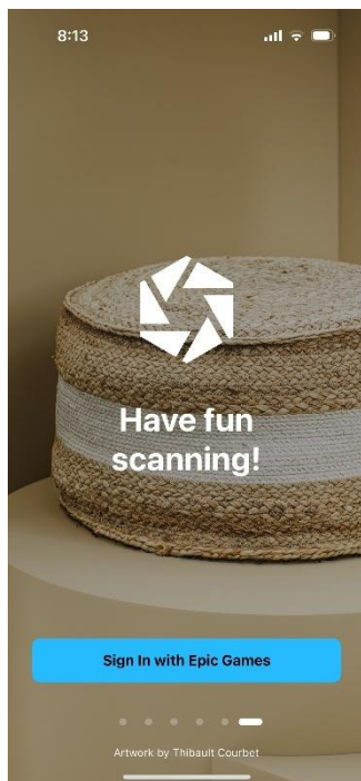
Obr. 1 Prihlásenie
