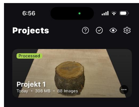
Obr. 25 Ukončenie spracovania
