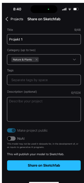
Obr. 29 Popis projektu
