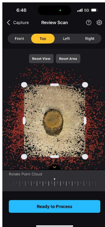
Obr. 20 Orezanie objektu
